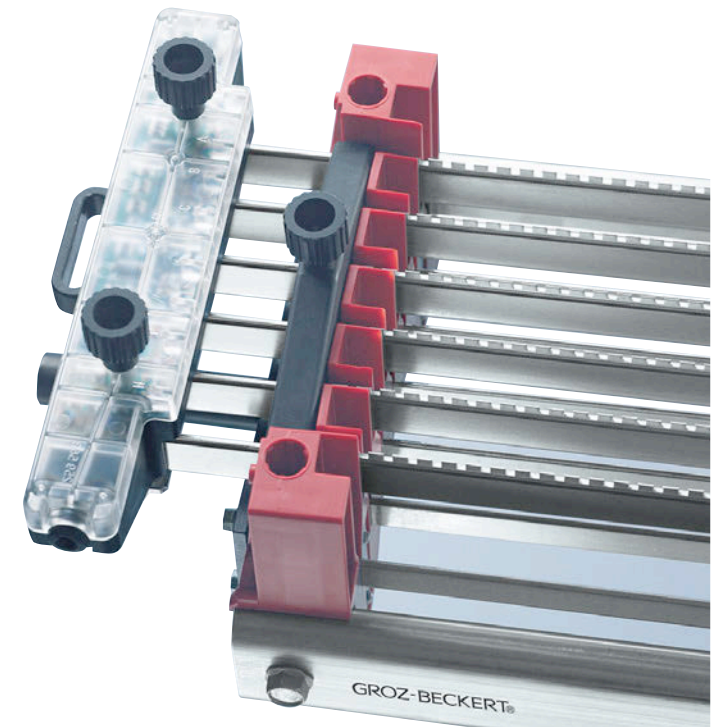
Kettfadenwächter 5600
